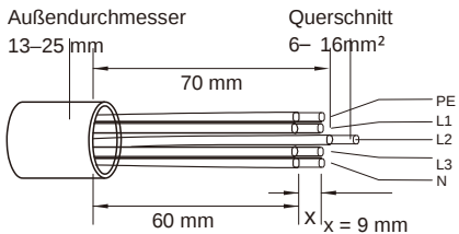
Abbildung 5.20 Abisolierter und entblößter Draht
