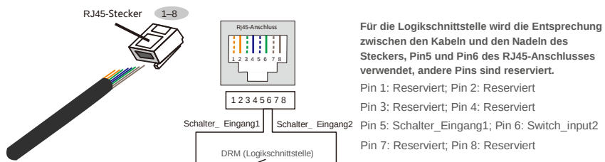
Abbildung 5.31 Abisolieren der Isolationsschicht und Anschluss an RJ45-Stecker
