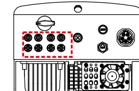
Abbildung 5.18 Verbindung des Gleichstromsteckers mit dem Wechselrichter
