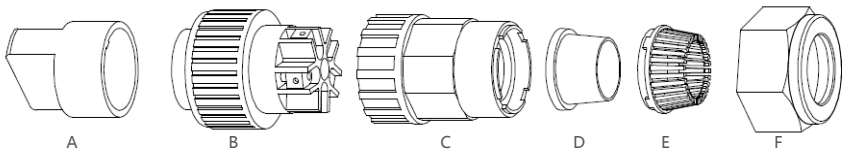
Abbildung 5.19 Wechselstromstecker
