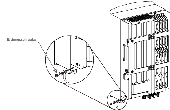
Abbildung 5.10 Befestigtes Kabel
