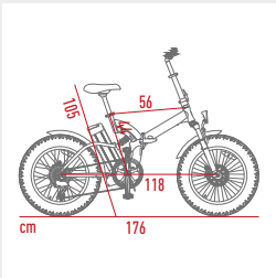
Dimensioni e-bike
