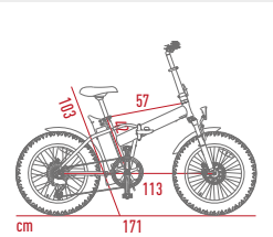
Dimensioni e-bike
