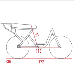
Dimensioni e-bike
